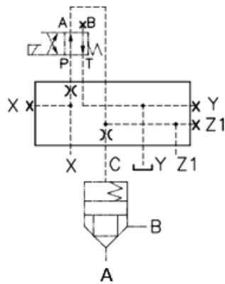
H9-LC*DEA-AZ1***
