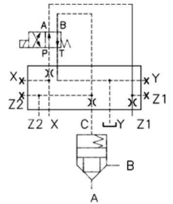
H9-LC*DEB-AZ1-BZ2**
