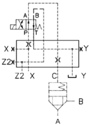
H9-LC*DEA-BZ2**
