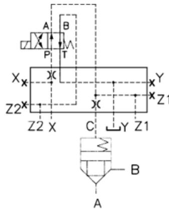
H9-LC*DEA-AZ1-BZ2**
