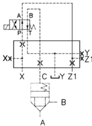
H9-LC*DEB-AZ1**
